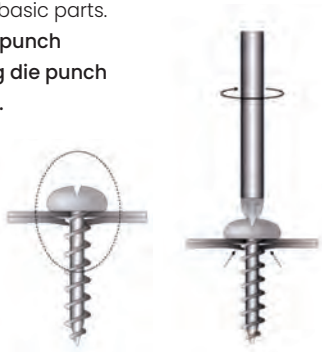
2 - Embossing Die Punch
